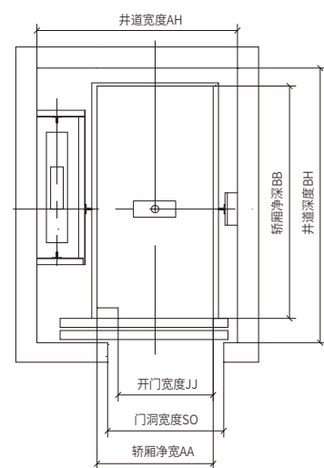
井道平面布置图
